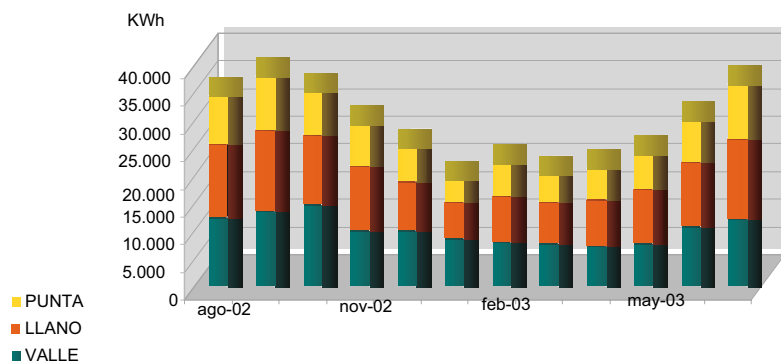
CURVA DE CARGA ELÉCTRICA EN DH4
